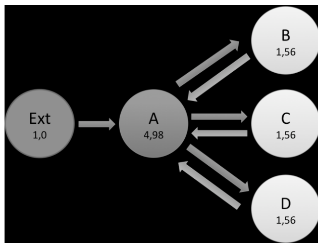
Figure 35. Calcul du PageRank (2)
